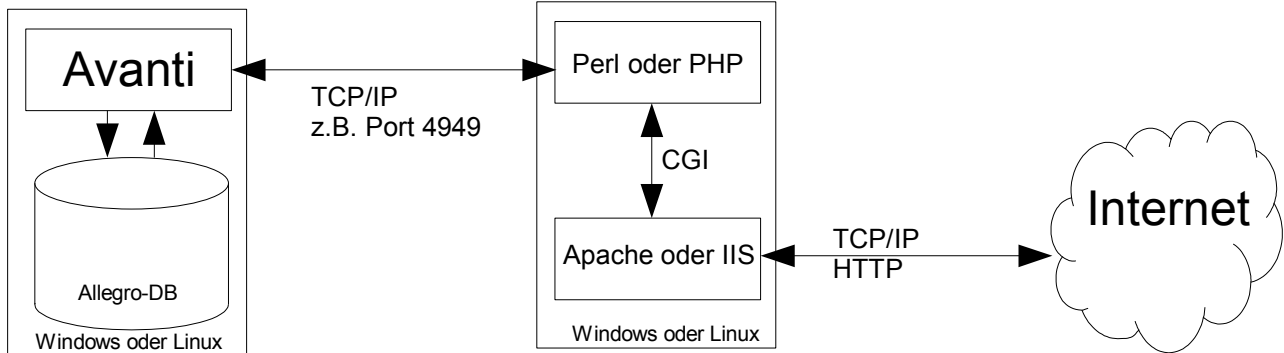
Avanti auf DB-Server
